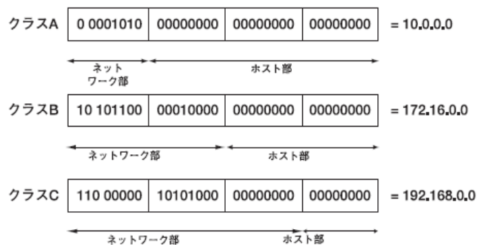
P.99 図3.9 IPアドレスのクラス(正)
